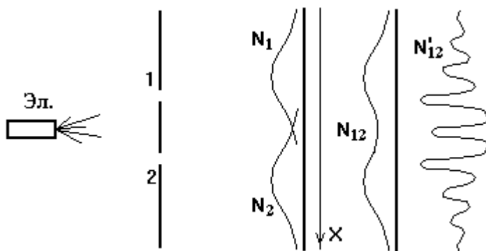
Рис.4. Корпускулярно-волновой дуализм
