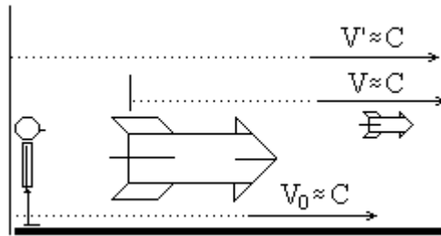
Рис. 2. Релятивистское правило сложения скоростей
